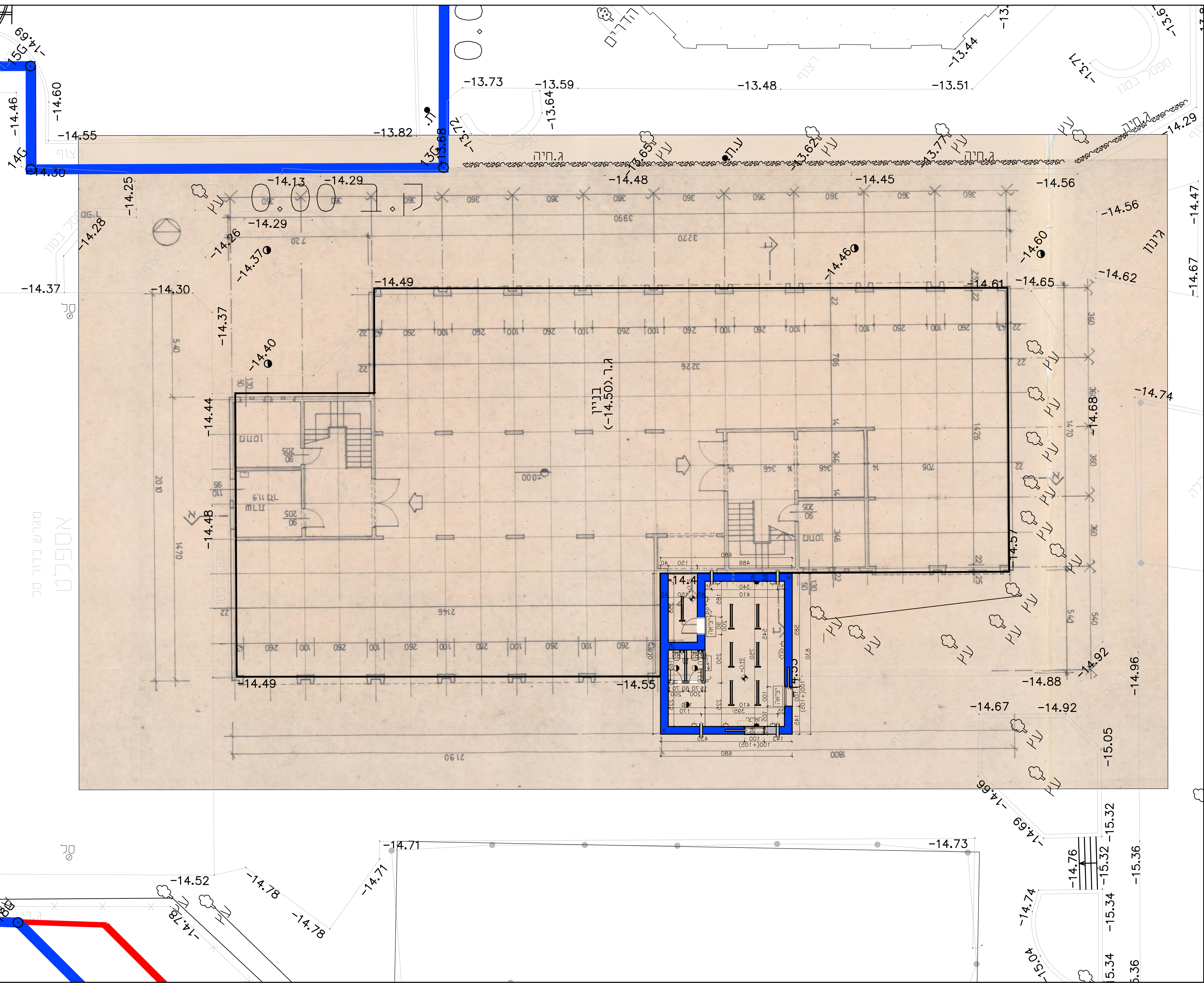
תכנית העמדה 1:100
