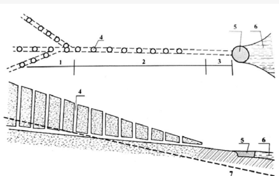
איור 1. תכנית וחתך סכמתיים במערכת בארות-מנהרה: (1) מנהרה החודרת לאופק מי-תהום; (2) מנהרה ותעלה מקורה המוליכות מים; (3) תעלה פתוחה; (4) פירים; (5) ברכת אגירה; (6) שטח מעובד; (7) אופק מי תהום.
