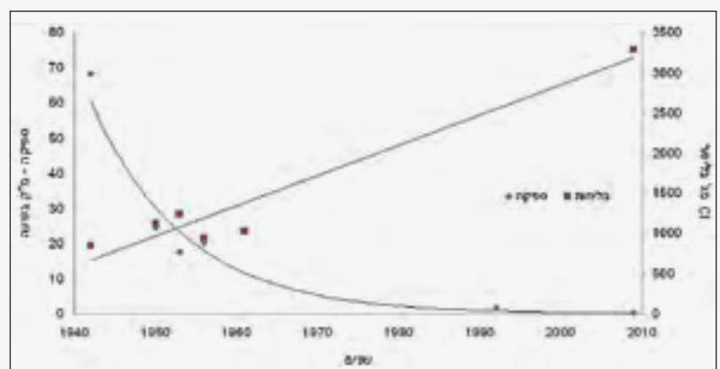
מעיינות בערבה - שינויים עם הזמן עין תמר - שינויים בספיקת המים וברמת המליחות בשנים 1944-2010
